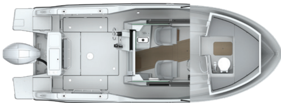
Nedre dekk
